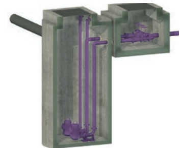
Ersatzneubau Pumpwerk und Pumpendruckleitung, PW Wisbach, Fällanden: 3D-Modell Pump- und Armatureschacht. Der Schacht wurde aus vorgefertigten Schachtbauteilen erstellt. Die gesamte Pumpendruckleitung wurde ersetzt und in grösserer Dimension neu ausgeführt.
