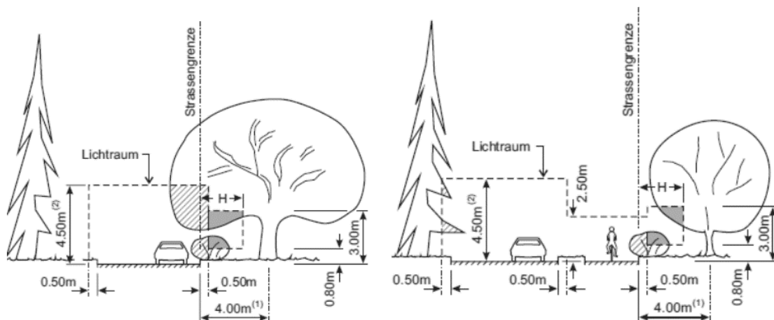
Abbildung 1: Lichtraumprofil
