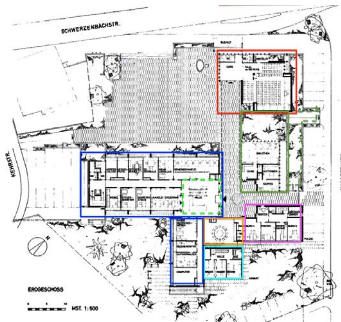
Gemeindehausplatz, zentral gelegen im Gemeindehauskomplex
